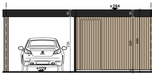
ACHTERGEVEL
