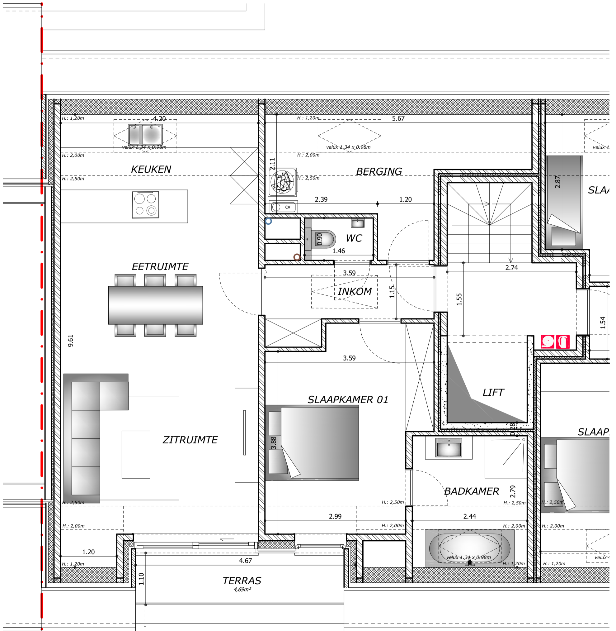
lot 06_APP.02.01 - Oppervlakte: 79,94m 2 GRONDPLAN - 1/50
