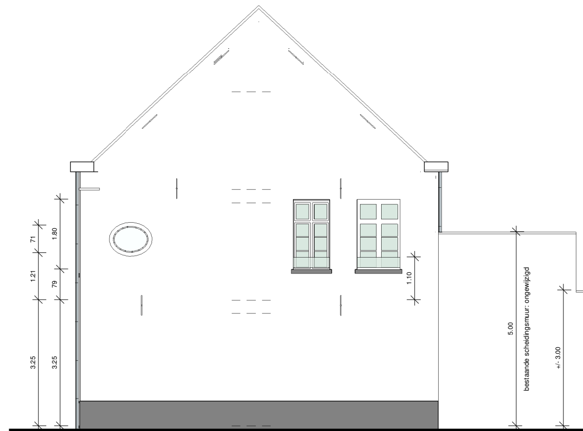
3 Zijgevel - Woning 4
