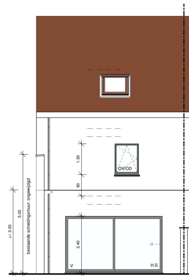
2 Achtergevel - Woning 4
